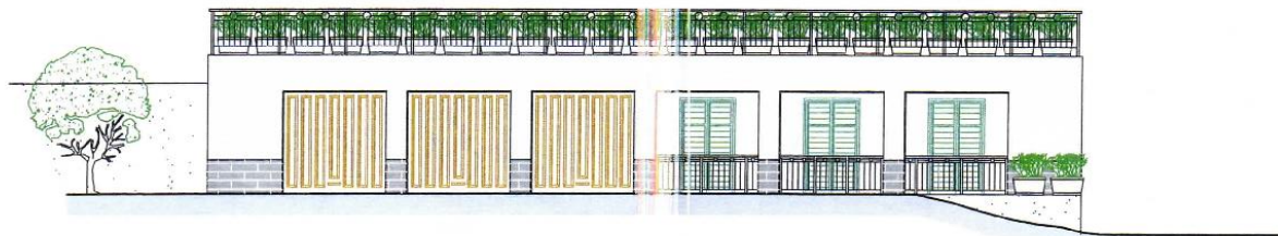
PROSPETTO FRONTALE
