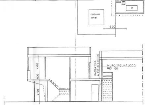
SEZIONE A A scala 1:100
